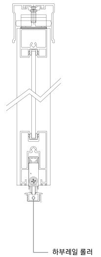
프레임설계 세부구조도
