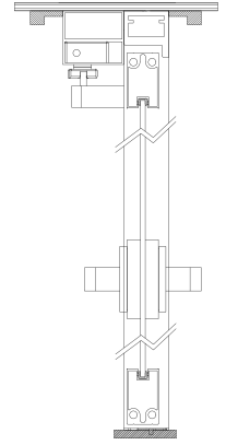
프레임설계 세부구조도
